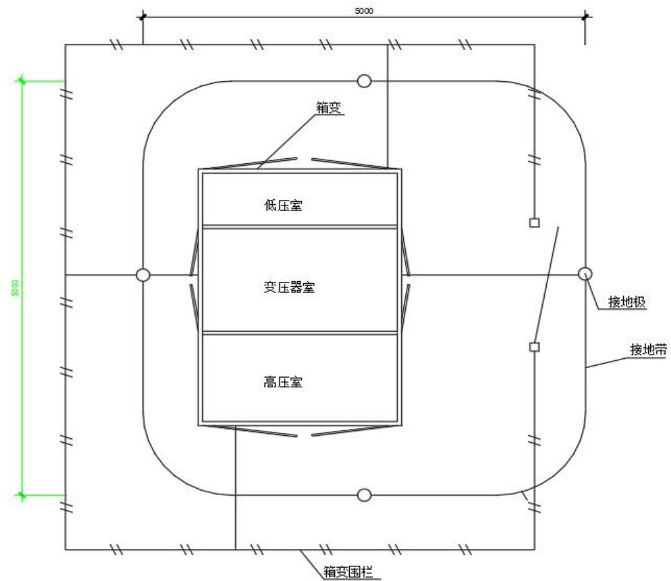
图 33. 箱变基础图（由设备厂家提供）
