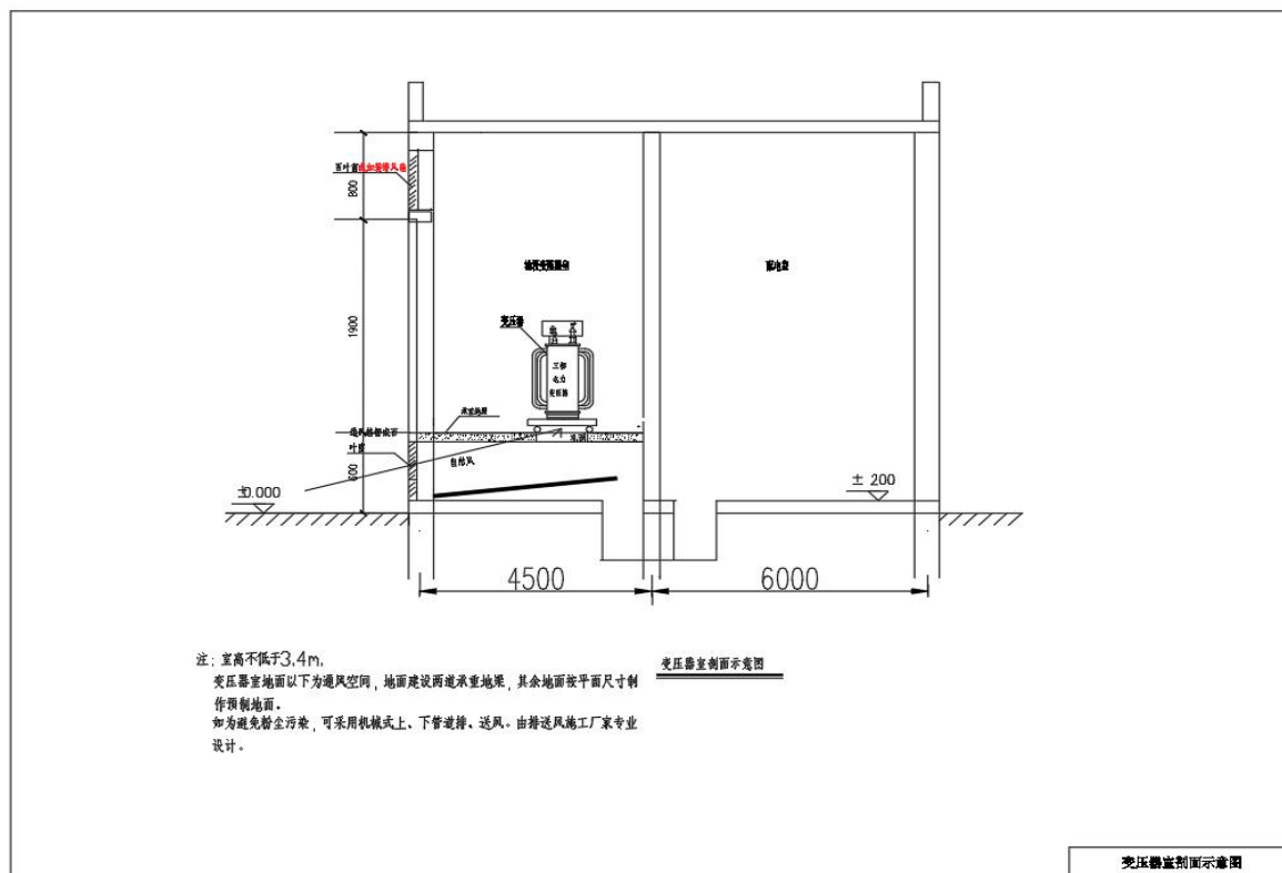
图 38. 变压器室剖面图
