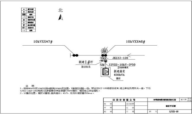
图 28. 路径平面图（含材料表）
