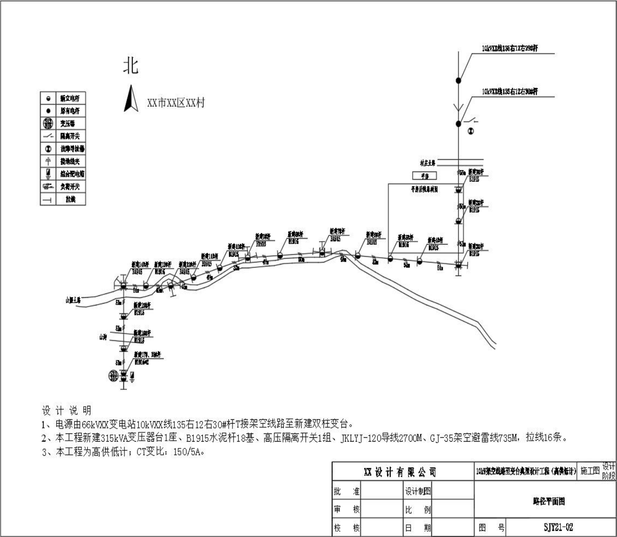
图 4. 路径平面图（含材料表）
