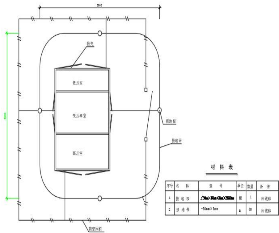
图 39. 配电室接地布置图
