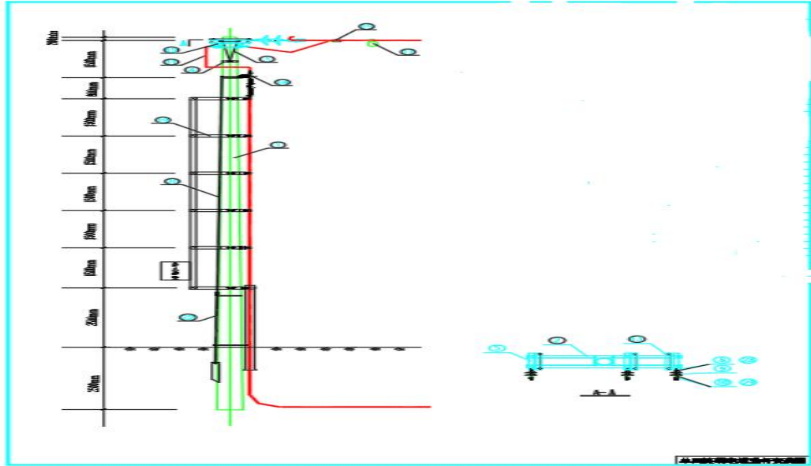
图 31. 电缆登杆图
