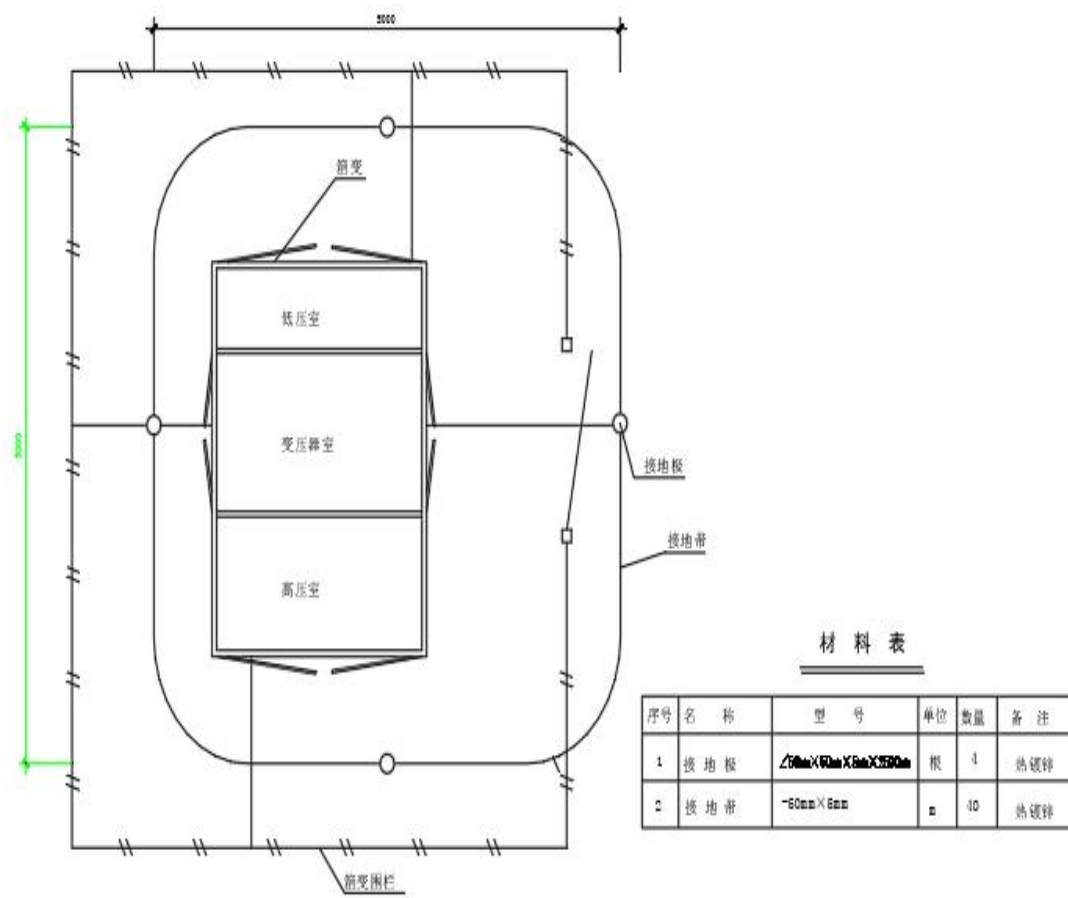
图 20. 配电室接地布置图
