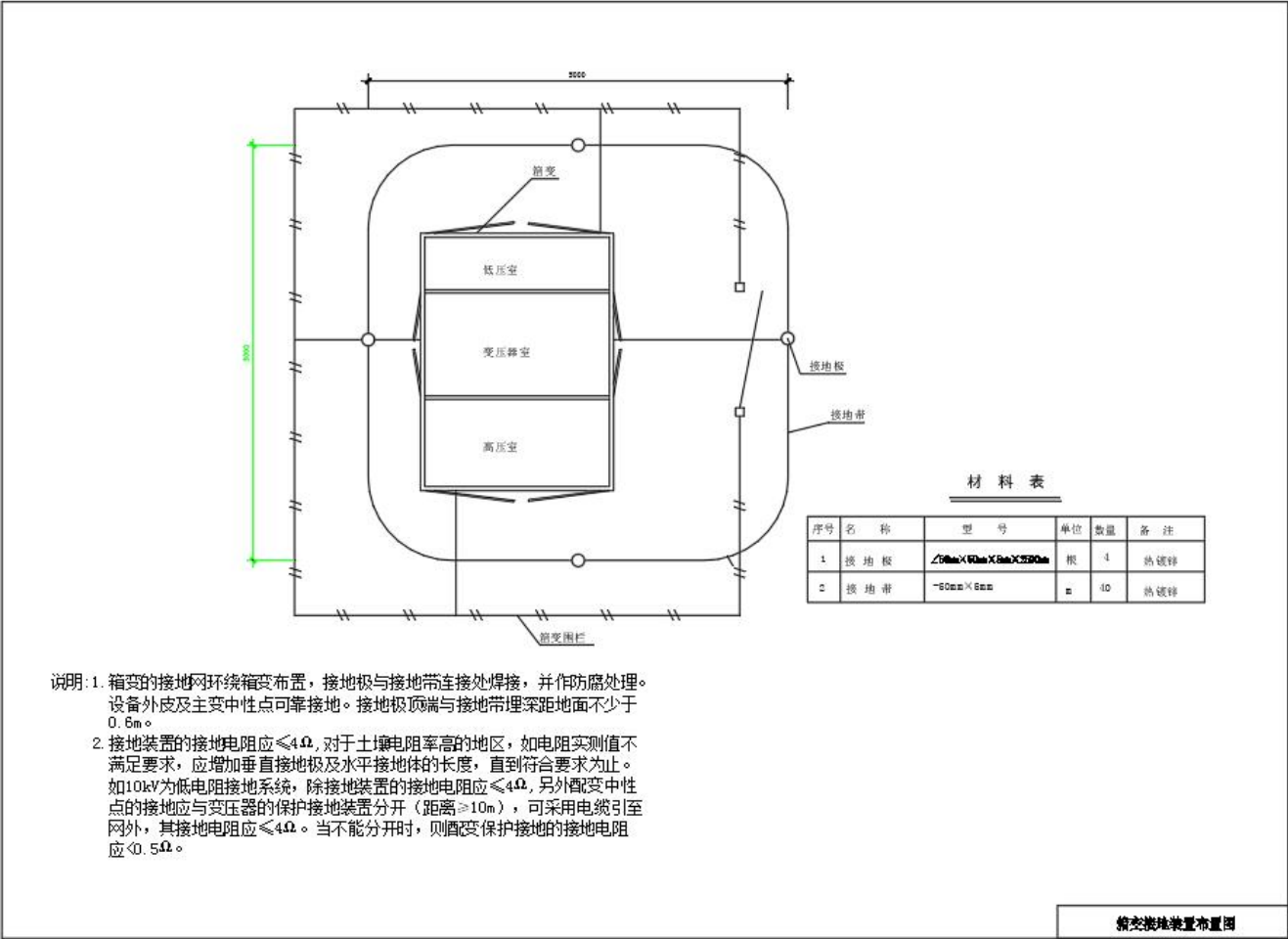
图 11. 箱变接地布置图
