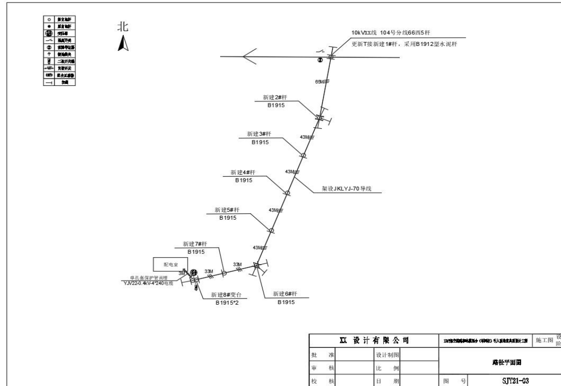
图 36. 路径平面图（含材料表）
