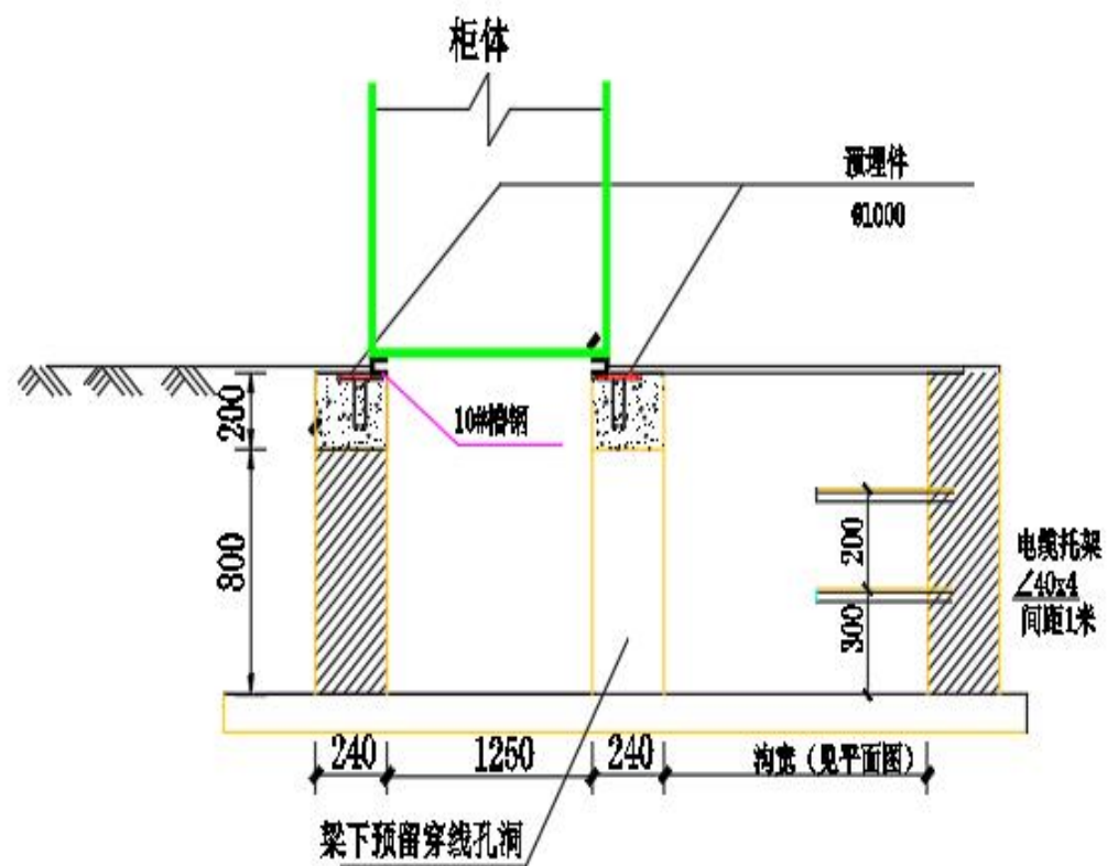
图 21. 配电室电缆沟布置图
