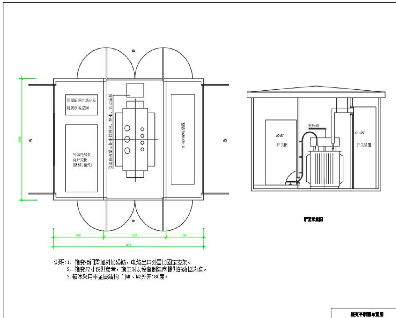
图 10 箱式变电站系统图
