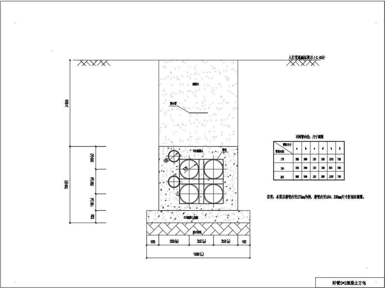
图 15. 排水沟剖面图
