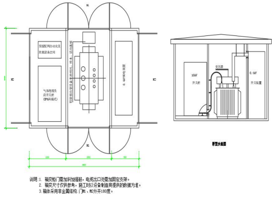
图 29. 箱式变电站系统图
