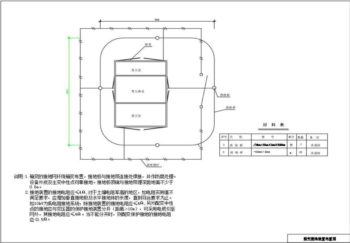
图 30. 箱变接地布置图
