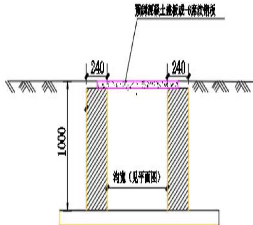
图 42. 电缆沟剖面图
