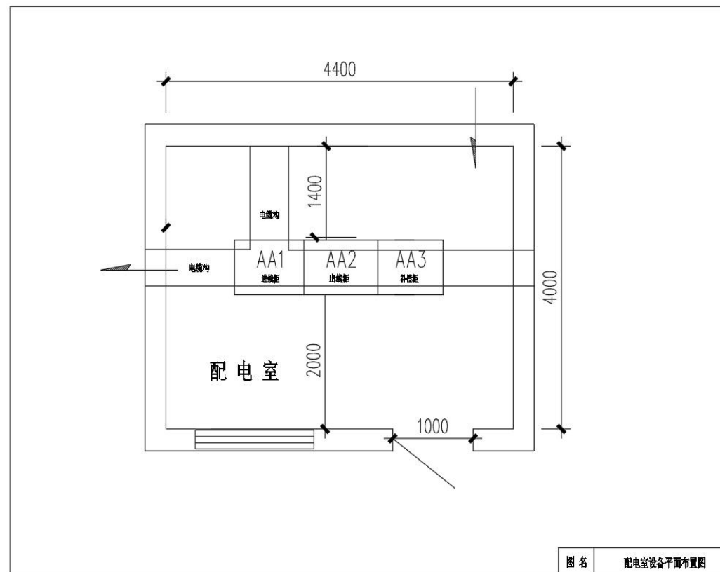
图 41. 配电室布置图
