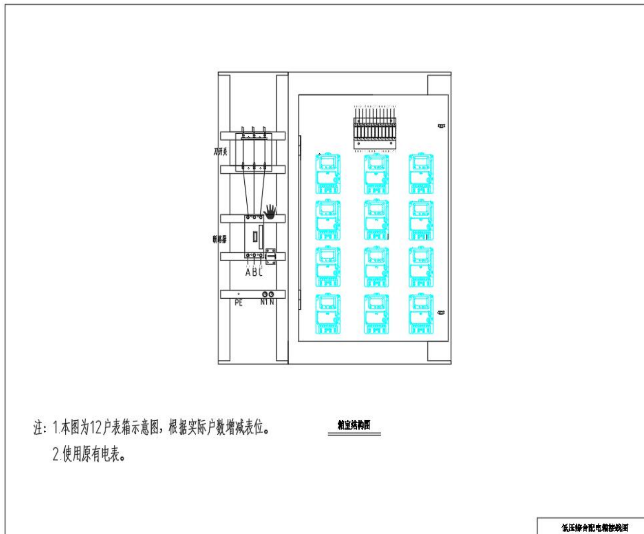
图 8. 低压综合配电箱接线图
