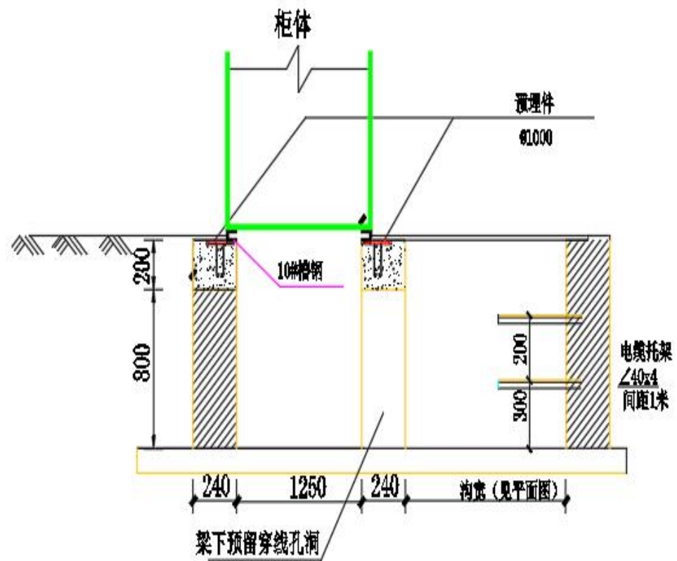
图 40. 配电室电缆沟布置图
