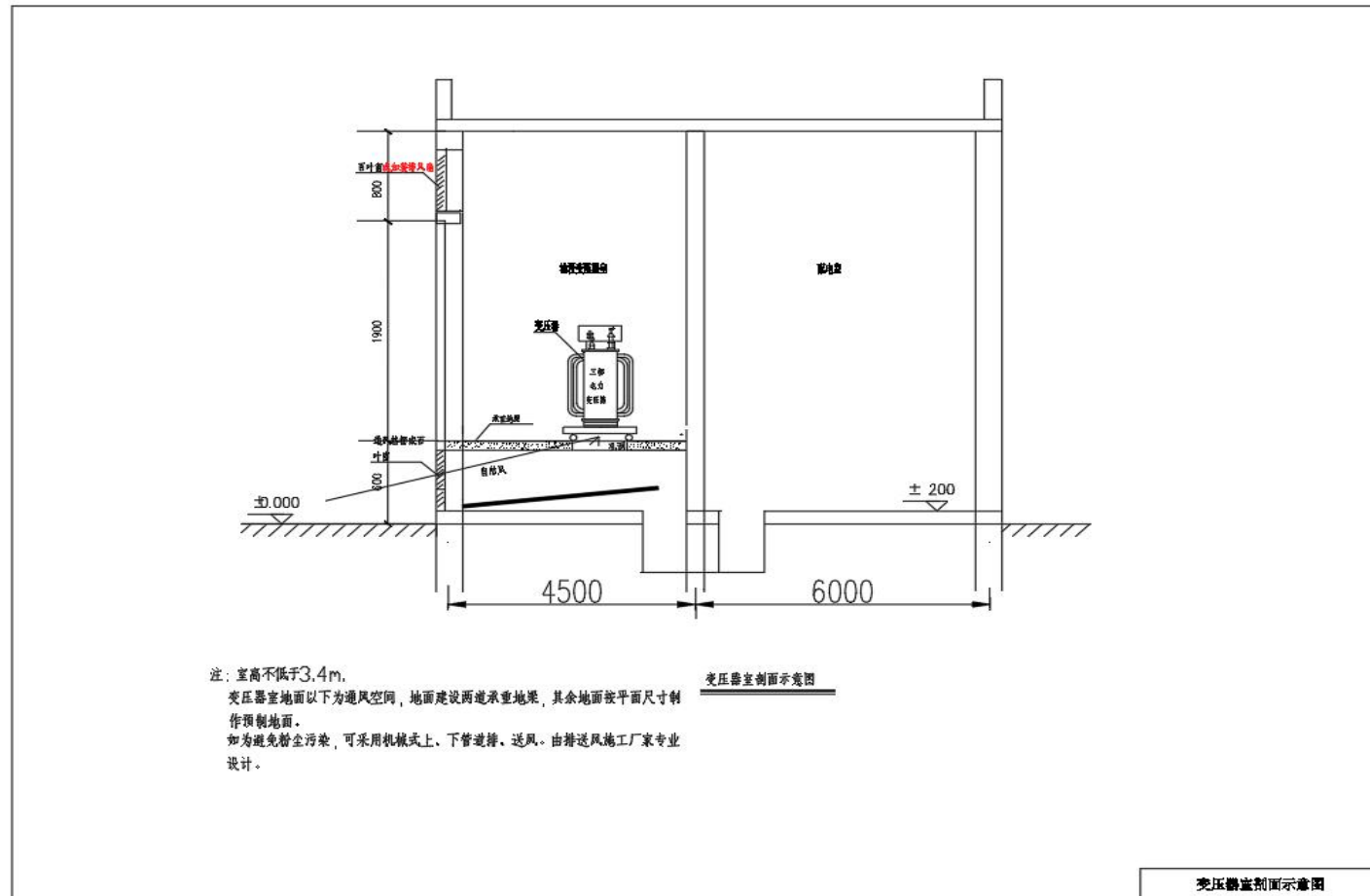
图 19. 变压器室剖面图
