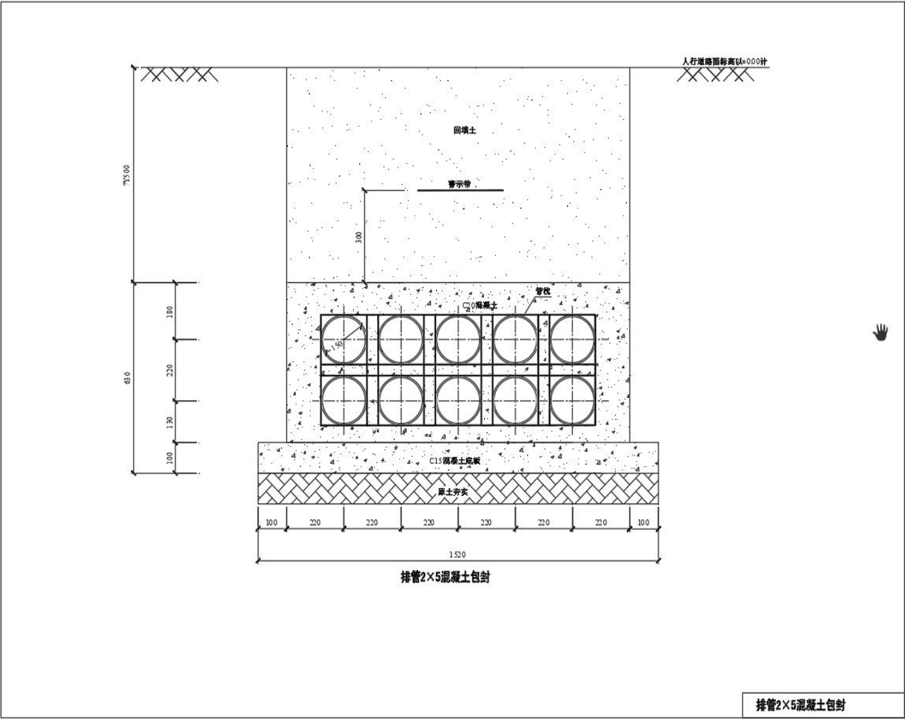
图 3. 电缆沟剖面图
