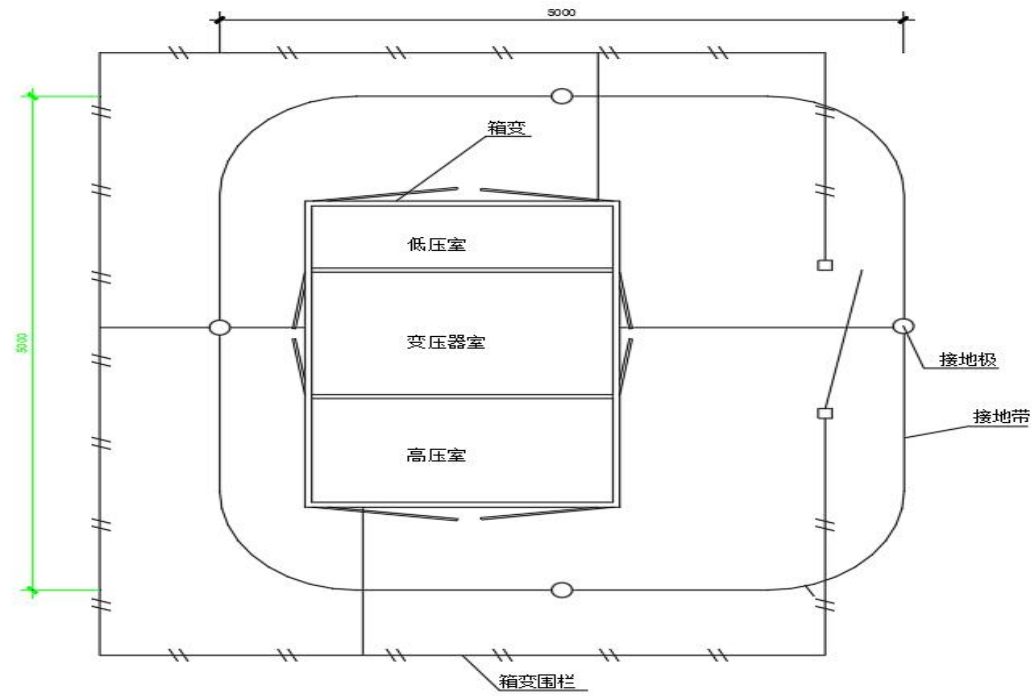
图 14. 箱变基础图（由设备厂家提供）
