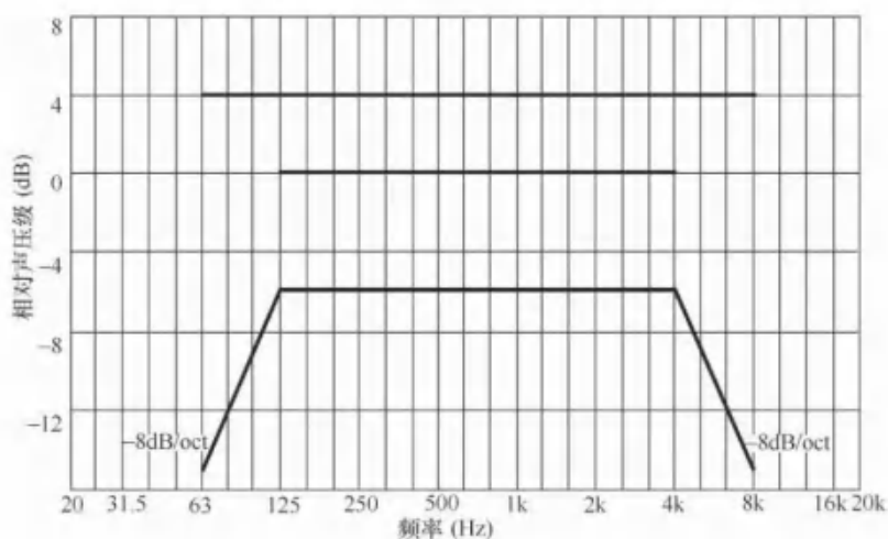
图 20.8.18-2 二级会议扩声系统传输频率特性
