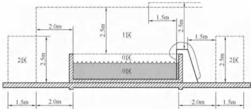
图 D-2 地面上游泳池和戏水池的区域尺寸（侧视图） 注：最后确定的区域尺寸需视现场中墙和隔板的位置而定。
