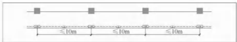
图 13.6.5-2 直行疏散走道疏散照明布置示意
