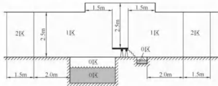
图 D-1 游泳池和戏水池的区域尺寸（侧视图） 注：最后确定的区域尺寸需视现场中墙和隔板的位置而定。
