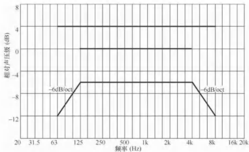
图 20.8.18-1 一级会议扩声系统传输频率特性
