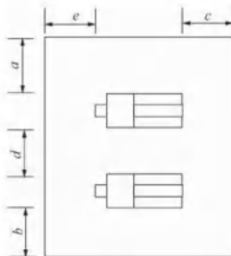
图 6.1.4 机组布置
