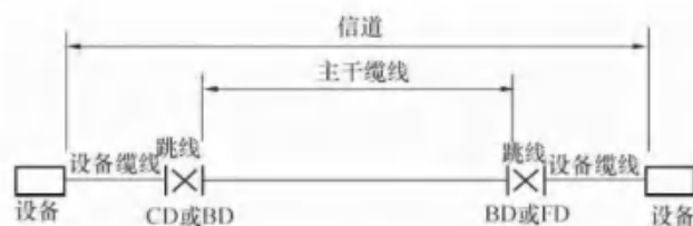
图 21.2.5-2 干线子系统线缆划分
