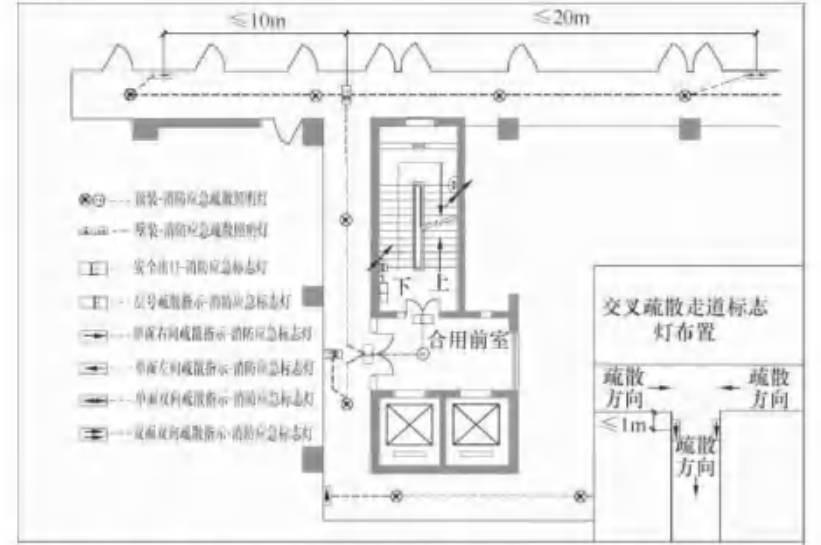
图 13.6.5-1 疏散走道、防烟楼梯间及前室疏散照明布置示意
