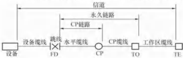
图 21.2.5-1 配线子系统线缆划分
