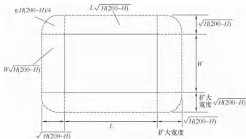
图 B. 1. 3 建筑物的等效面积
